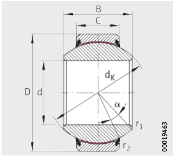
GE..-FW-2RS ELGOGLIDE®
