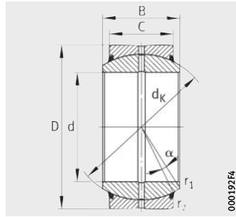
GE..DO-2TS Steel/steel
