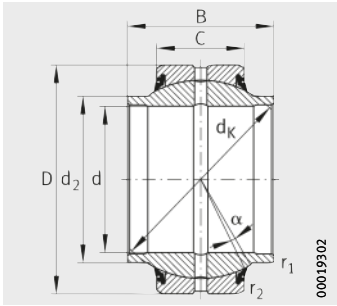
GE..-HO-2RS Steel/steel
