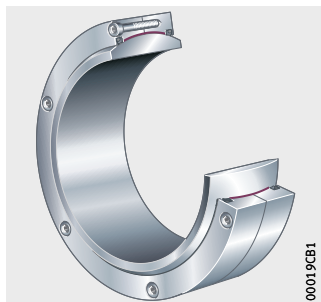
GE..-DW-2RS2
